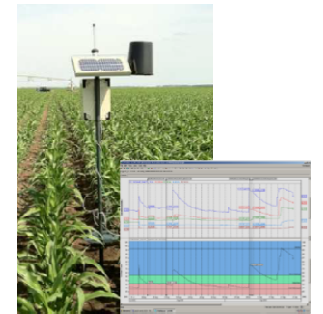
Etat hydrique du sol (Tensiomètre)
